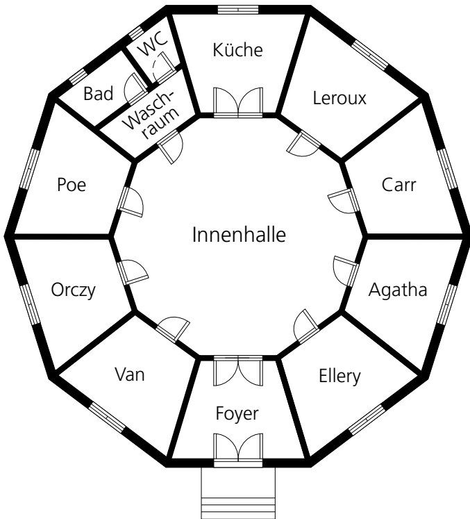
Abb. 1 Grundriss Dekagon-Haus
